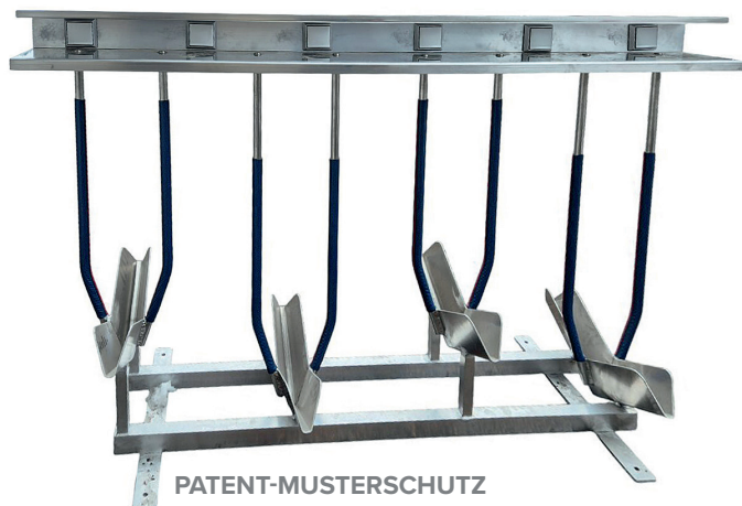
Fahrradständer mit Steckdosen für E-Bikes
